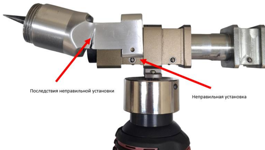
Рис. 2 Неправильная установка расширительного адаптера на аксиальном прессе
